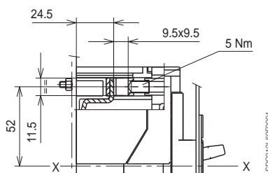
Front for copper/aluminum cables - FC CuAl 50 mm 2
